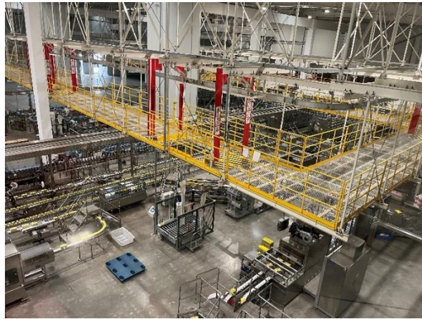
維他奶工廠自動分配懸掛系統
