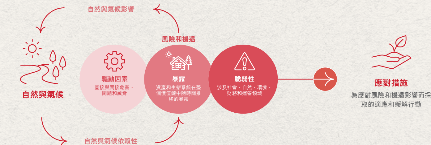
气候与自然相关联系示意图
